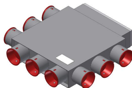
Rozdělovací box s devíti nástavci
