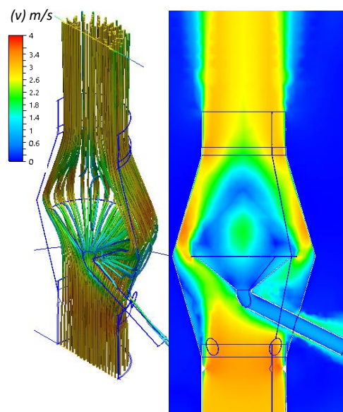
Rychlost proudění vzduchu ve výfuk. hlavici
