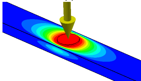
Oblasti nejvyššího průhybu
